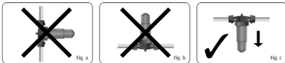
FörfilterPLUS och filtersystemet ska alltid installeras vertikalt, som på figur C.
